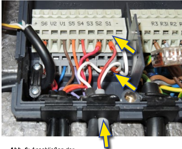
Abb. 6: Anschließen der Zirkulationstemperatursonde.
